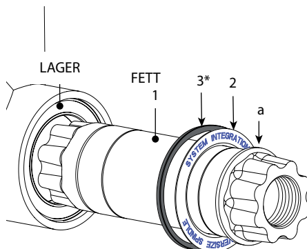
NICHTANTRIEBSSEITE
