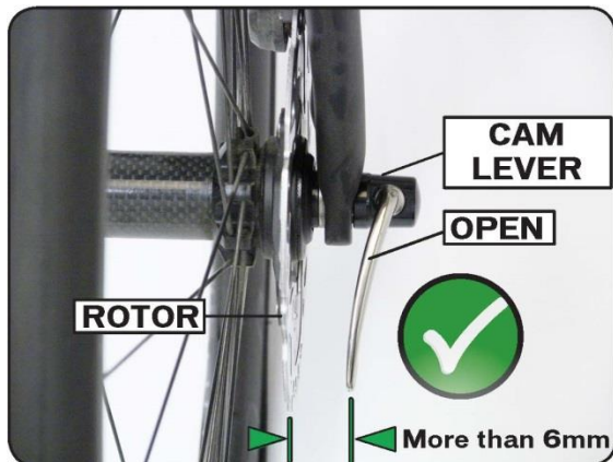
Abbildung 2. Schnellspanner mit richtigem Abstand zwischen Hebel und Scheibenbremse.
