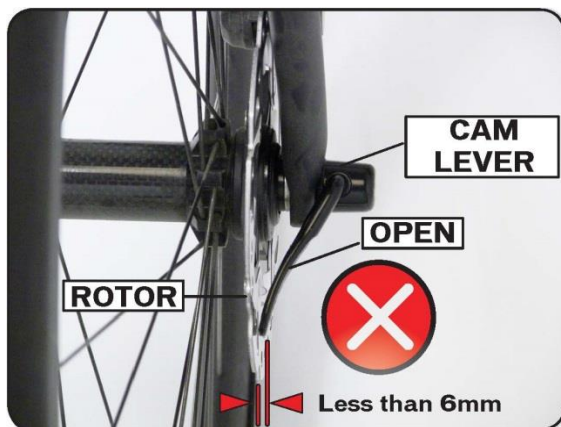
Abbildung1. Schnellspanner mit Gefahr des möglichen Kontakts von Hebel und Scheibenbremse.
