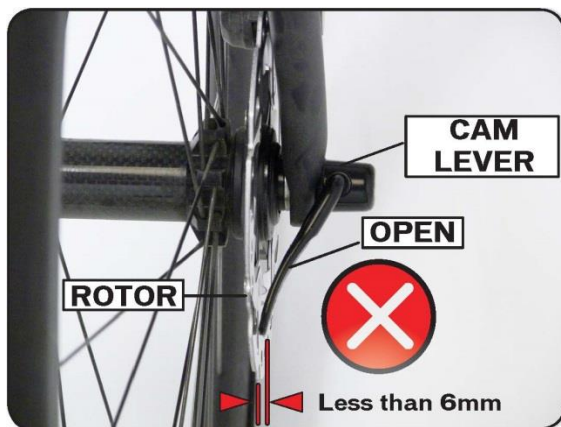
图1. 快拆杆存在潜在性的机会，会碰到碟盘
