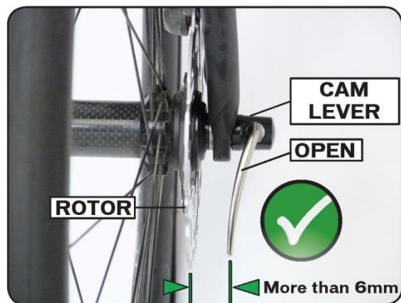
图2. 快拆杆跟碟盘有足够的间隙
